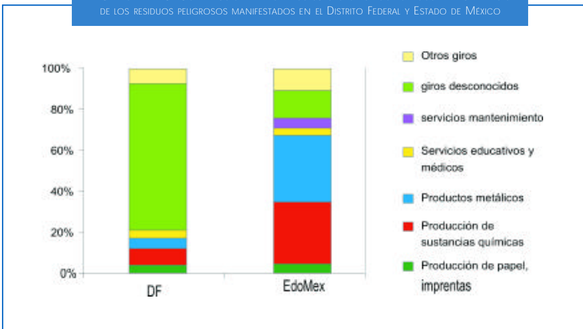
GRÁFICA 2.26. CONTRIBUCIÓN DE DISTINTOS SUBSECTORES ECONÓMICOS A LA GENERACIÓN DE LOS RESIDUOS PELIGROSOS MANIFESTADOS EN EL DISTRITO FEDERAL Y ESTADO DE MÉXICO
