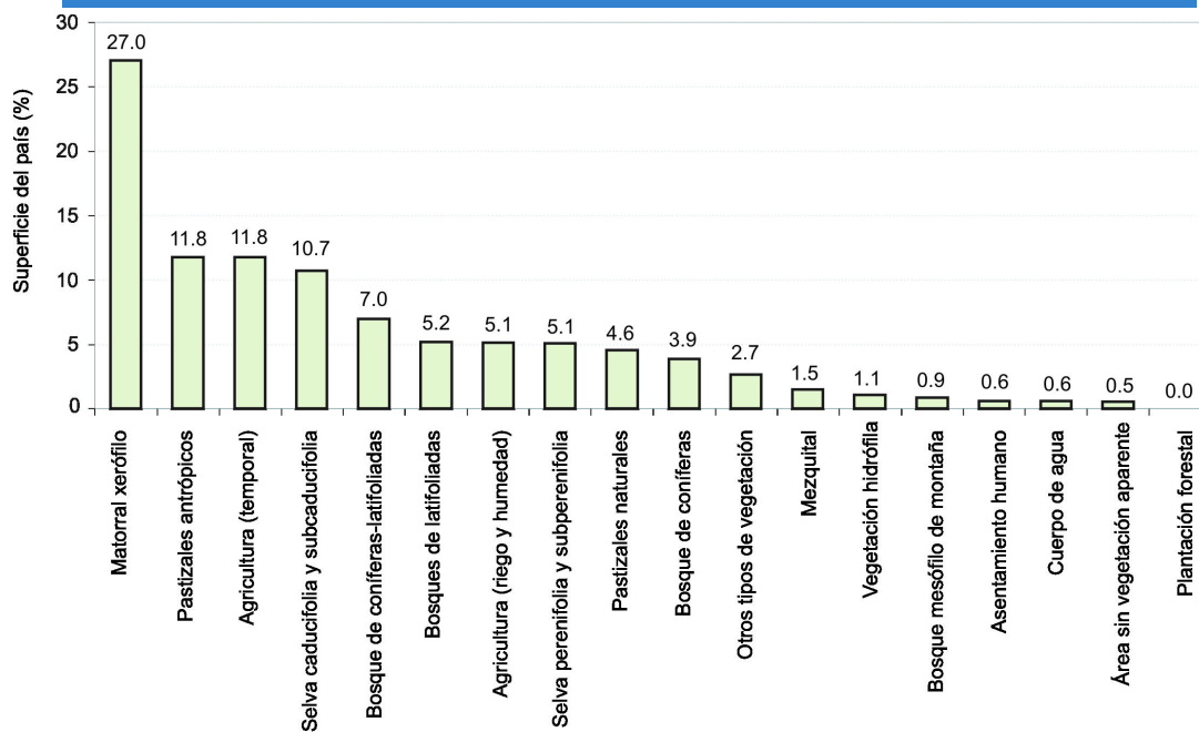
GRÁFICA 2.43. SUPERFICIE RELATIVA DE LOS TIPOS DE VEGETACIÓN Y USO DEL SUELO EN EL AÑO 2000
