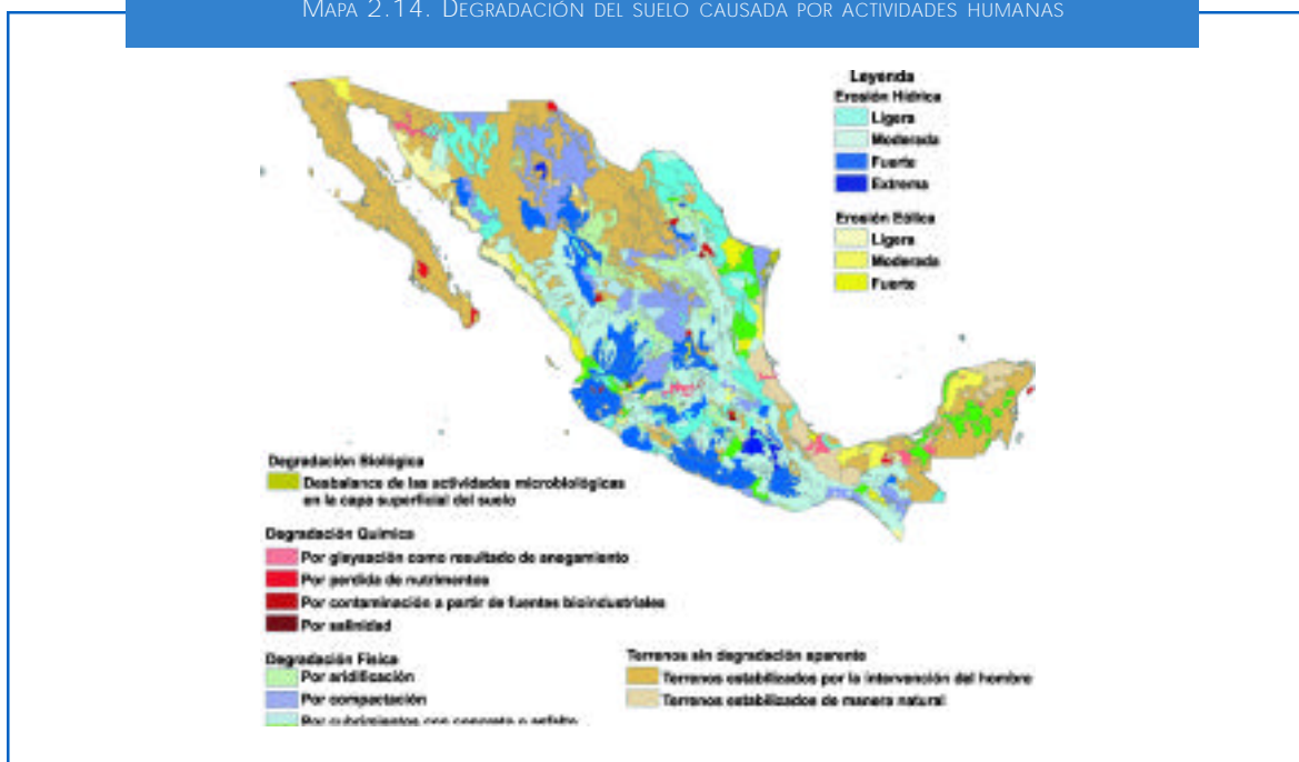
MAPA 2.14. DEGRADACIÓN DEL SUELO CAUSADA POR ACTIVIDADES HUMANAS
