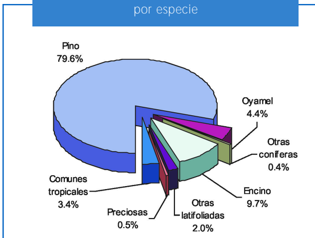
Gráfica 2.34 Producción nacional maderable por especie
