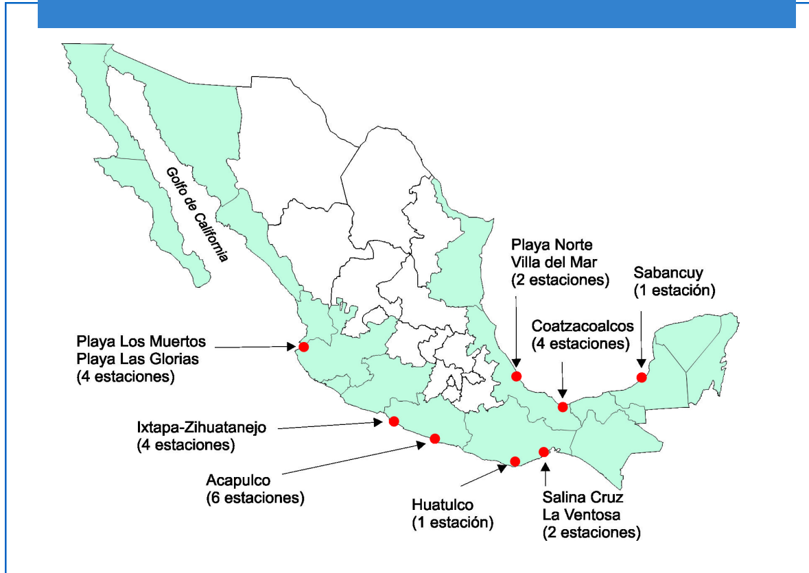
MAPA 2.12. ESTACIONES DE LA RED NACIONAL DE MONITOREO DE LA CALIDAD DEL AGUA EN ZONAS COSTERAS
