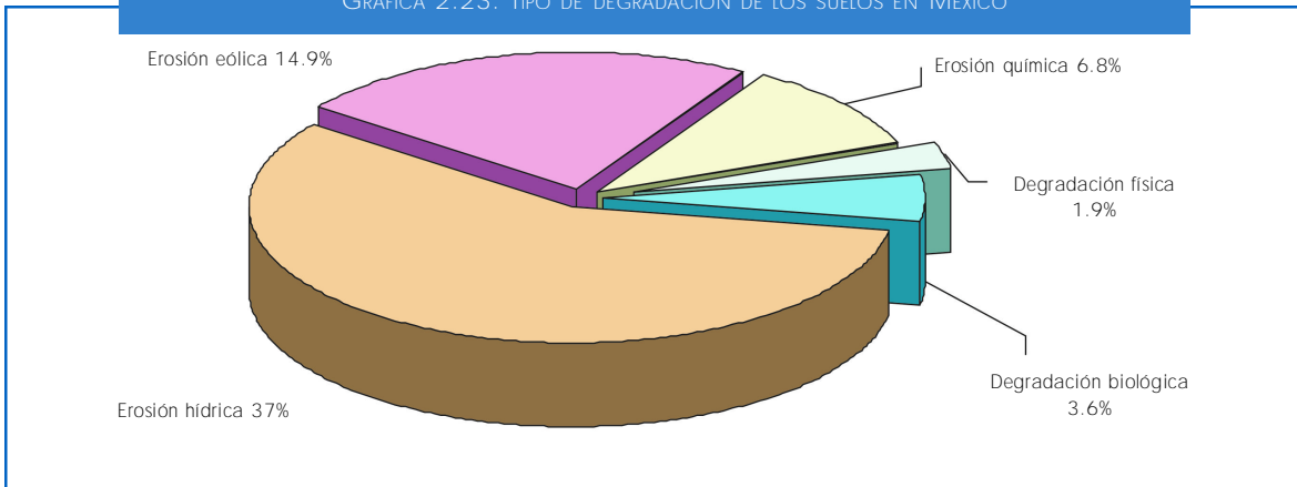
GRÁFICA 2.23. TIPO DE DEGRADACIÓN DE LOS SUELOS EN MÉXICO
