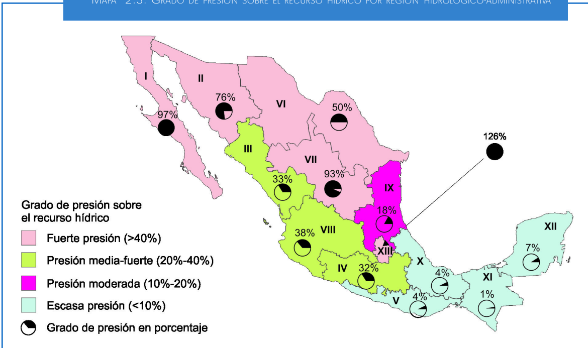
MAPA 2.3. GRADO DE PRESIÓN SOBRE EL RECURSO HÍDRICO POR REGIÓN HIDROLÓGICO-ADMINISTRATIVA *
