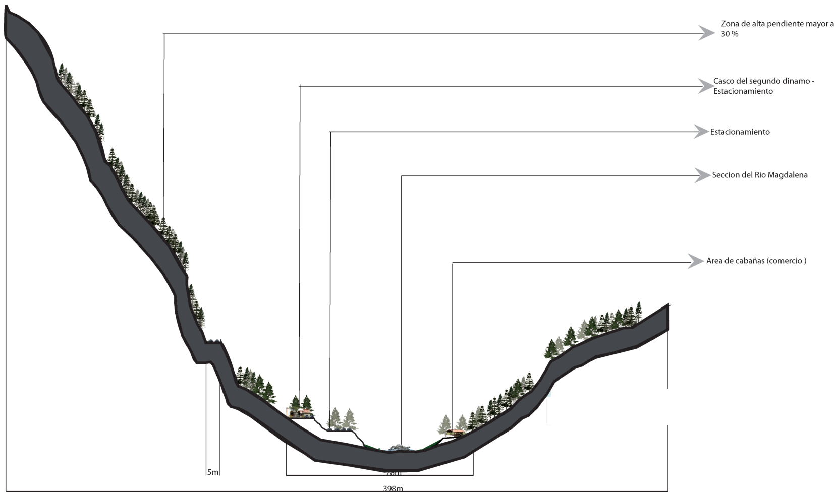
A-A' Corte transversal de la zona inmueble y comercio del 3er Dinamo Sección 3. SC3-A-A'
