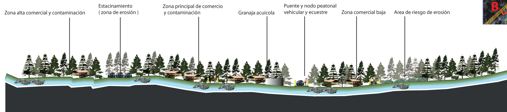
B-B' Corte longitudinal 2 de la zona de inmueble y comercio del 3er Dinamo Sección 12. SC12-B-B'
