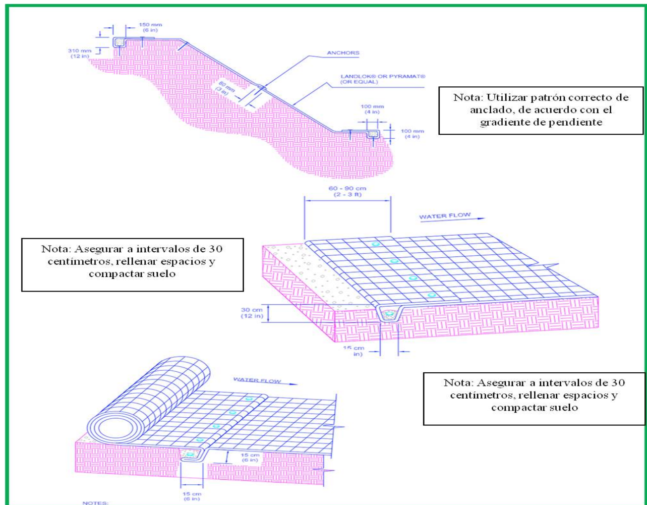
Fig. 4. Se ilustran los pasos para la colocación de geomallas en taludes erosionados.
