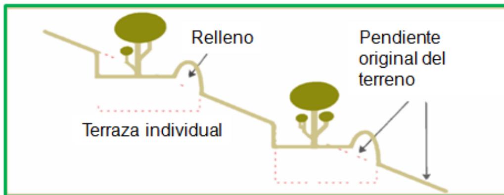
Fig. 43. Esquema de terrazas individuales.
