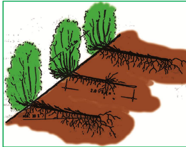
Fig. 40. Construcción de lechos de ramaje de setos vivos.
