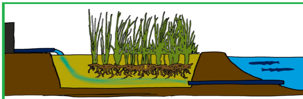
Fig. 20. Esquema de colocación de tubos en el humedal.
