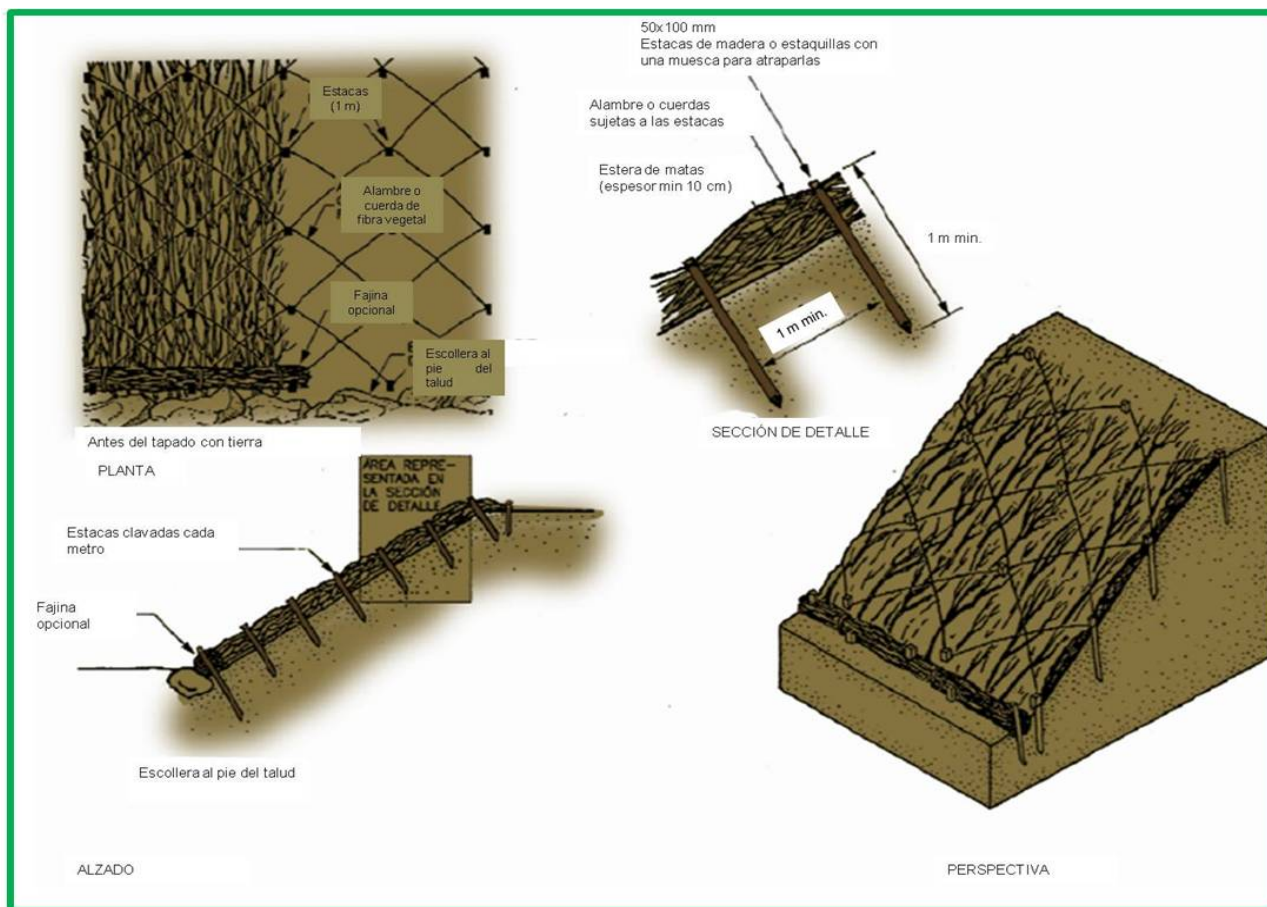
Fig. 10. esquema de instalación de las esteras marginales.
