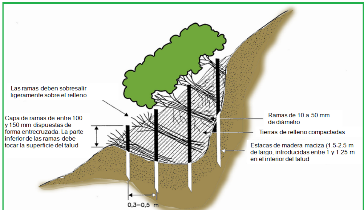
Fig. 31. Esquema de instalación de paquetes de matorral.
