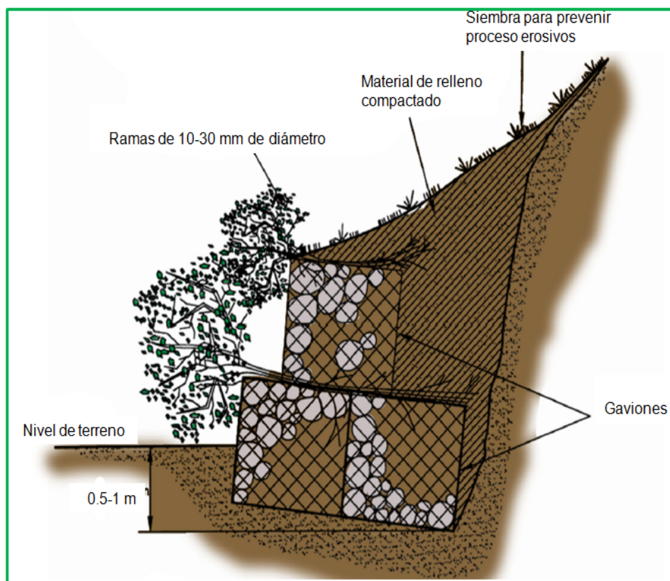
Fig. 42. Esquema de colocación de estaquillas con pisos de gaviones.
