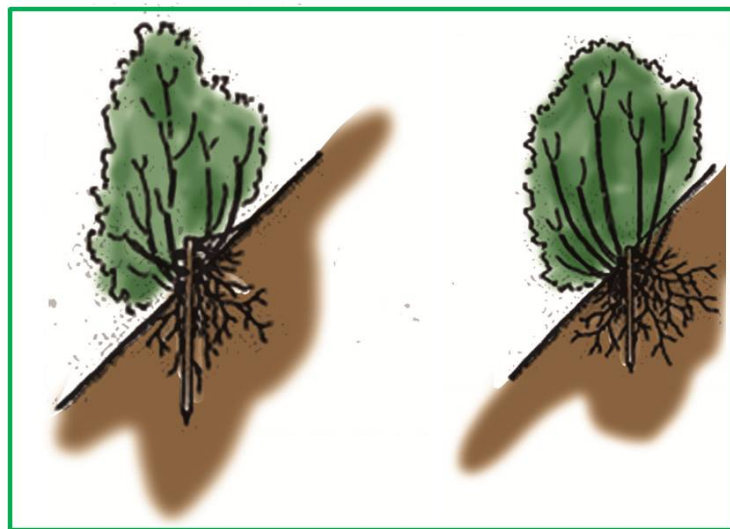
Fig. 34. Construcción de empalizadas trenzadas. A la izquierda, sobresaliendo del terreno. A la derecha, enrasadas.
