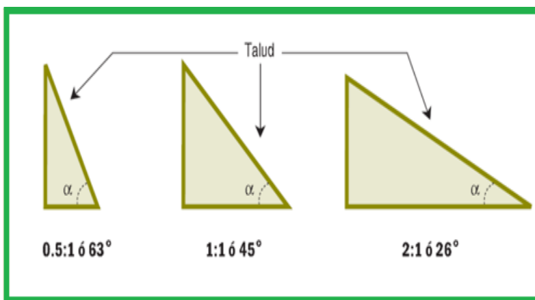
Fig. 5. Grados de inclinación para despalme de talud.
