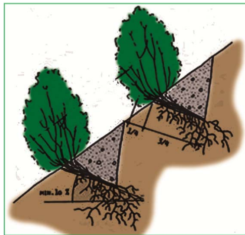
Fig. 38. Colocación de lechos de ramaje por debajo de cordones de vegetación.
