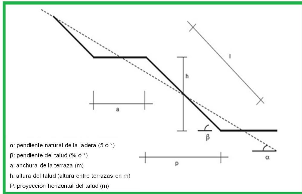
Fig. 13. Construcción de terrazas
