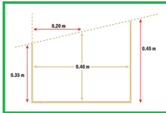
Fig. 22. Diferencia de profundidades de acuerdo con la pendiente.
