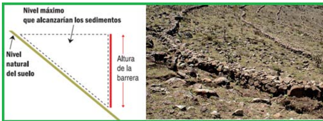
Fig. 8. Bardas construidas sobre curvas de nivel.
