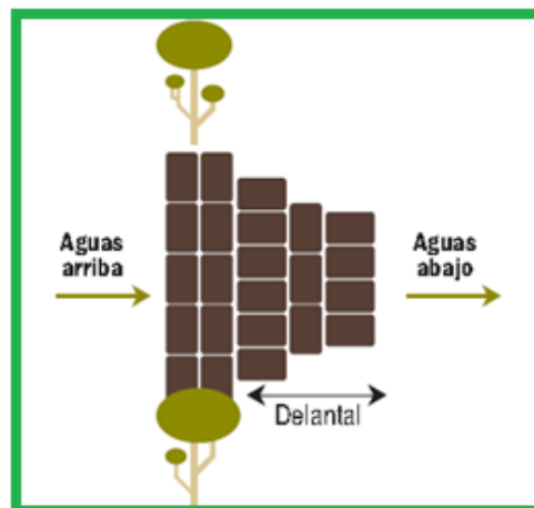
Fig. 24. Esquema para la colocación de delantal en las presas de geocostales.
