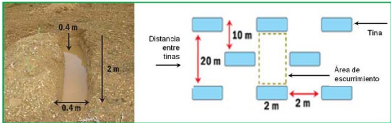
Fig. 21. Imagen con medidas promedio de una tina y esquema de posición de tinajas ciegas en tresbolillo.
