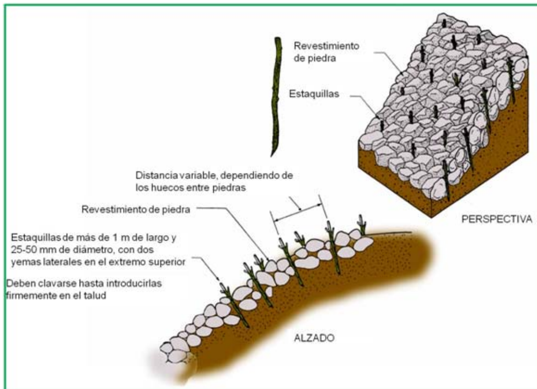
Fig. 41. Esquema de colocación de estaquillas en pedreras.
