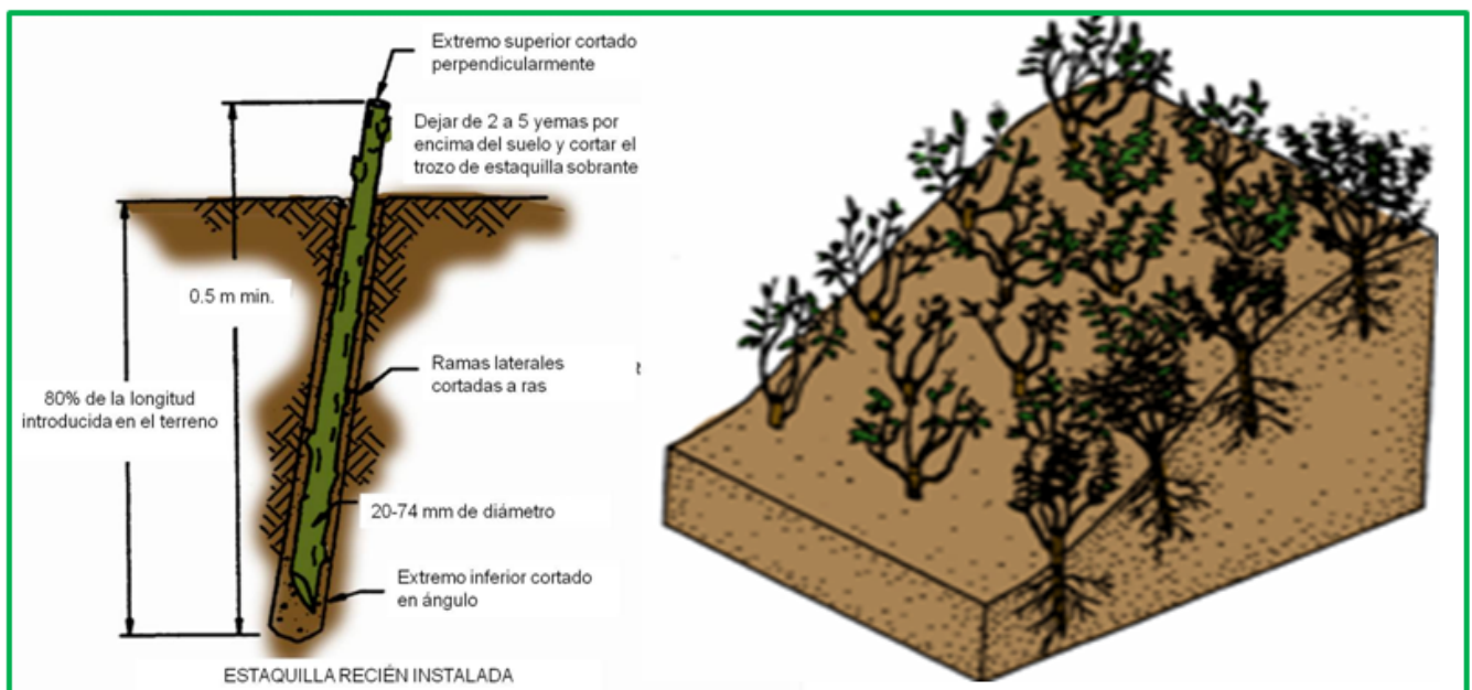
Fig. 30. Izquierda: Esquema de clavado de estaquillas. Derecha: Zona cubierta después de una estación de crecimiento.
