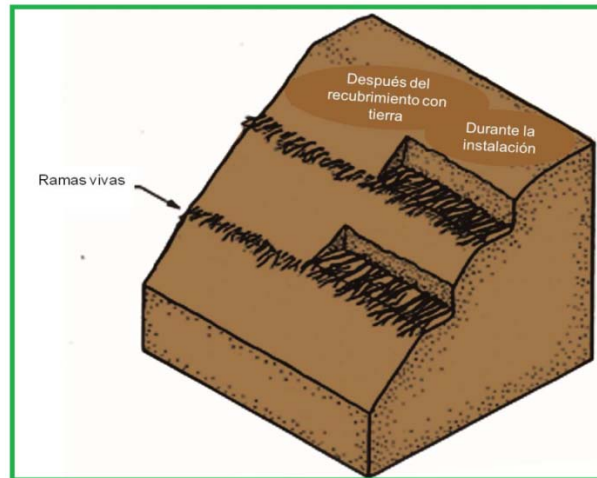
Fig. 39. Construcción de lechos de ramaje.
