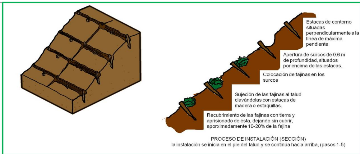
Fig.36. Fijación de fajinas de vegetación.
