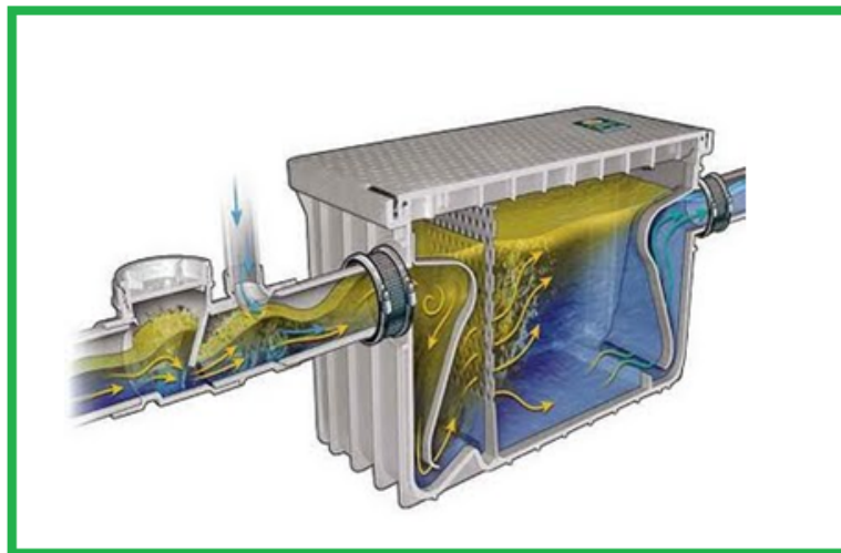
Fig. 16. Esquema de trampa de grasa.
