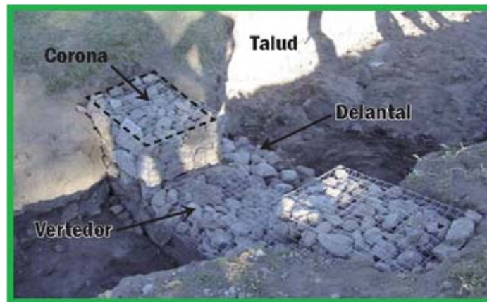
Fig. 29. Presa de malla ciclónica esquematizada.
