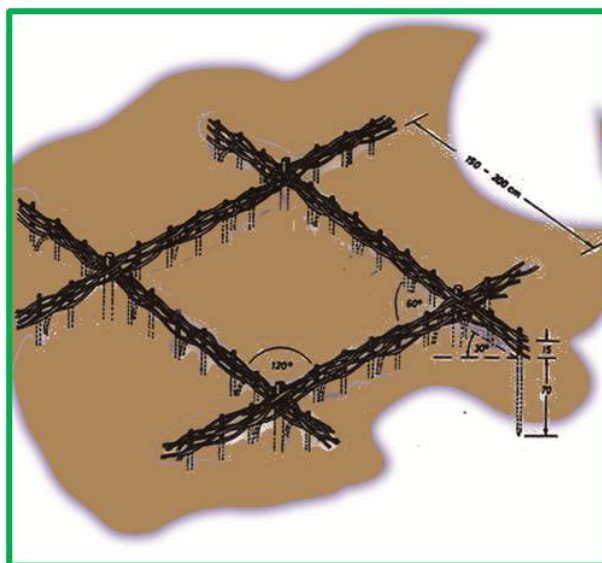
Fig. 38. Colocación en diagonal de empalizadas trenzadas.
