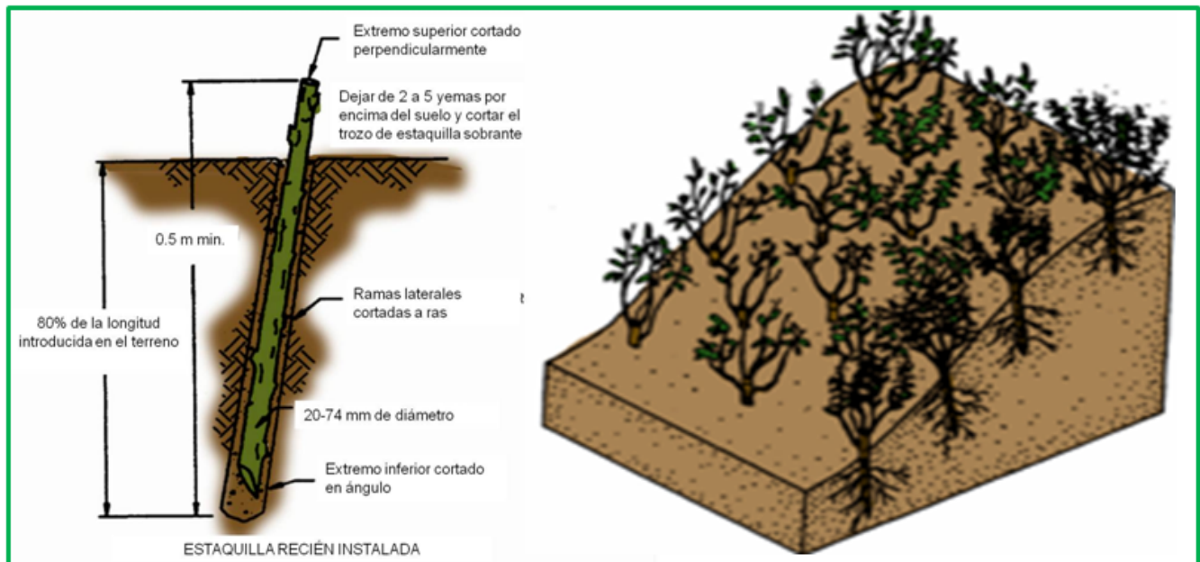
Fig. 33. Izquierda: Esquema de clavado de estaquillas. Derecha: Zona cubierta después de una estación de crecimiento.
