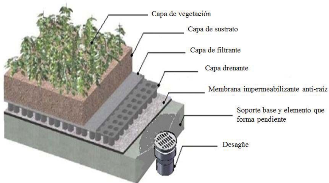
Figura 1. Componentes básicos de un sistema de naturación multicapa.
